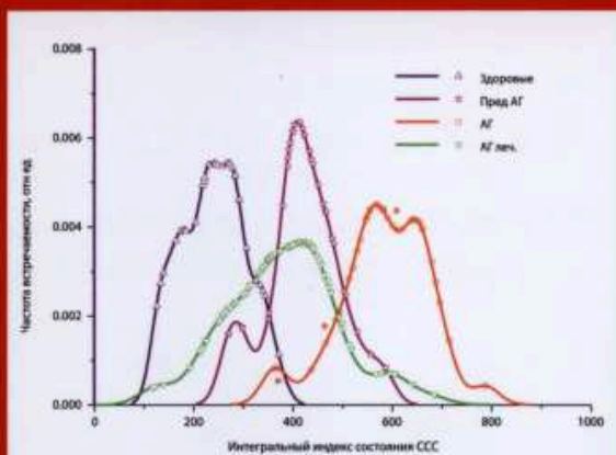
Рис. 4. График функции оценки плотности распределения интегрального индекса состояния сердечно-сосудистой системы (ССС).
